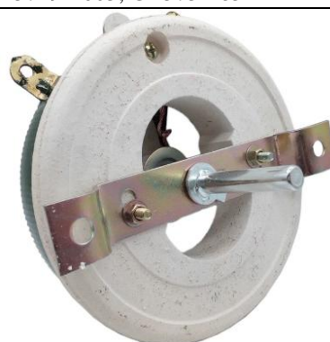
Figura 5 Reóstato BC1 de 500W. Fuente: [8]
